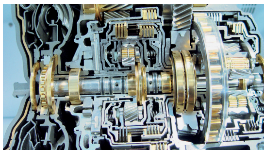
Construction mécanique
